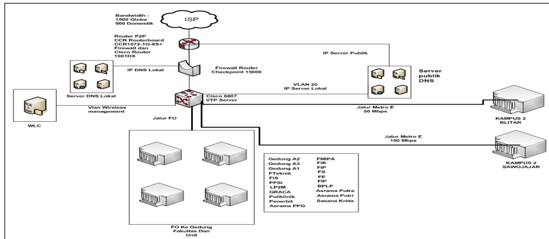
Gambar 2. Rencana Infrastruktur Jaringan Inti, Universitas Negeri Malang
